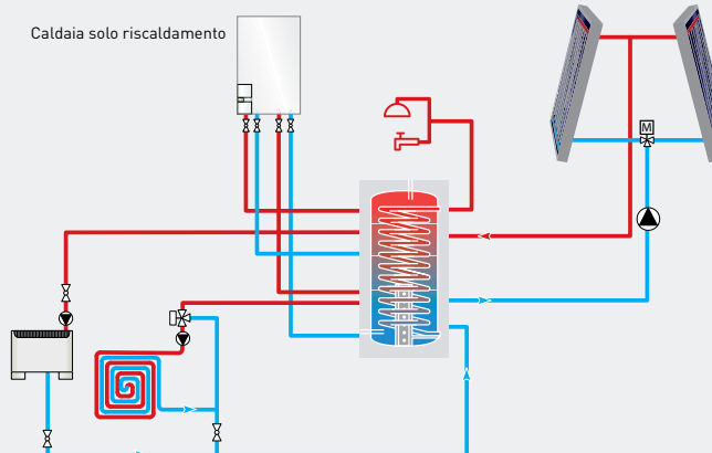
4 IMPIANTO SOLARE FORZATO DOPPIA FALDA CON PIPE IN TANK CON CALDAIA SOLO RISCALDAMENTO RISCALDAMENTO DIRETTO
