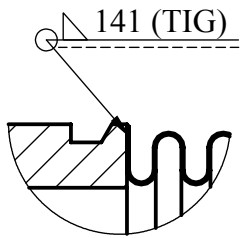
DETAY A ÖLÇEK 2 : 1
