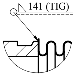
DETAY A ÖLÇEK 2 : 1
