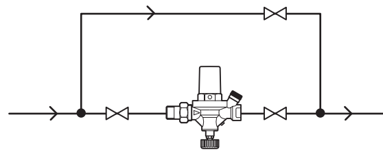
Schema d'installazione
