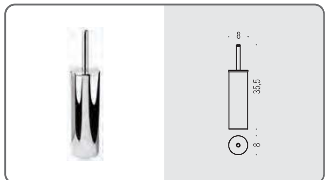
B2706 ○ Porta scopino d'appoggio Standing brush holder
